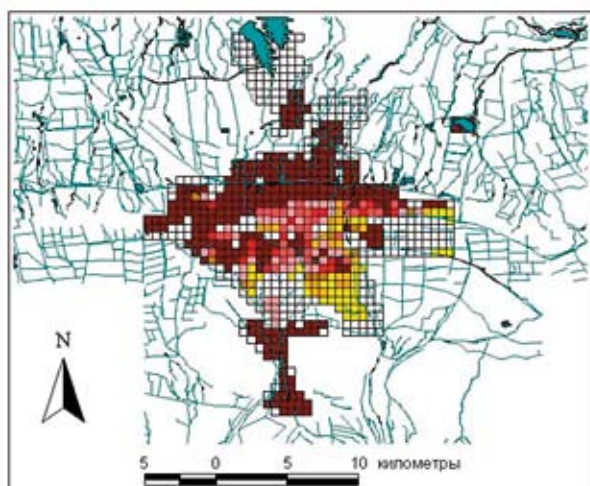
Bişekdäki ýaşaýs binalarynyň ähli görnüşleriniň seýsmiki ýumrulyşy
